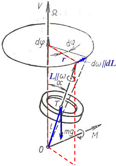
Obr. (2.5) 23. Precesní pohyb setrvačnicku vlivem
