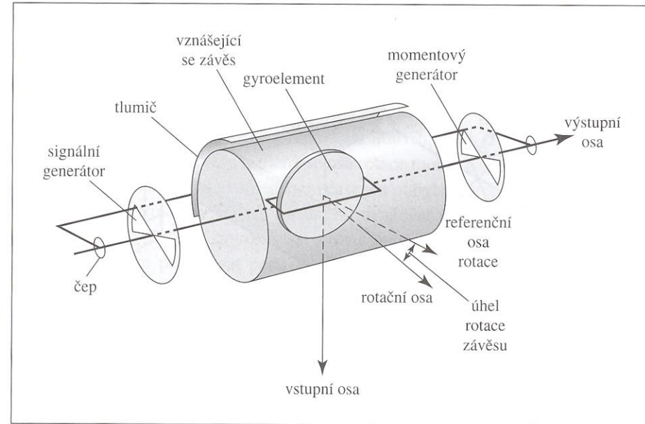
OBR. 4.11 Podrobné schéma integrujícího gyroskopu s jedním stupněm volnosti. Použit originální přednáškový diapozitiv.
