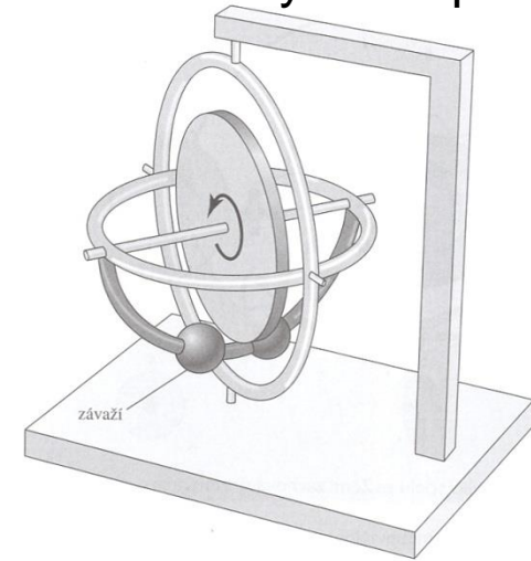
OBR. 4.6 Ukázka zatíženého gyroskopu, který má snahu udržovat rotační osu kolmou ke směru tíže.
