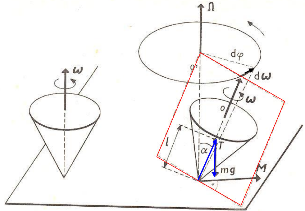
Obr. 4-20 Rotace vlčku na vodorovné podložce
