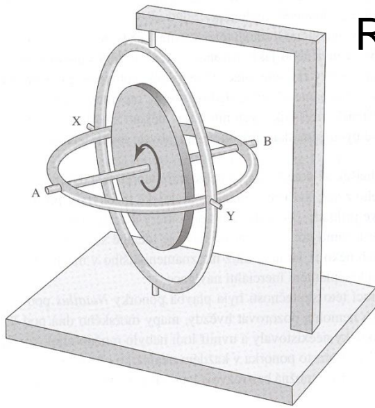
OBR. 4.1 Demonstrační gyroskop.
