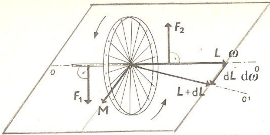
Obr. 4-17 Kinetická reakce setrvačníku
