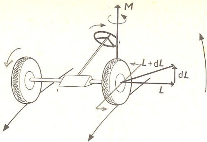
Obr. 4-18 Kinetická reakce kol automobilu při zatažení
