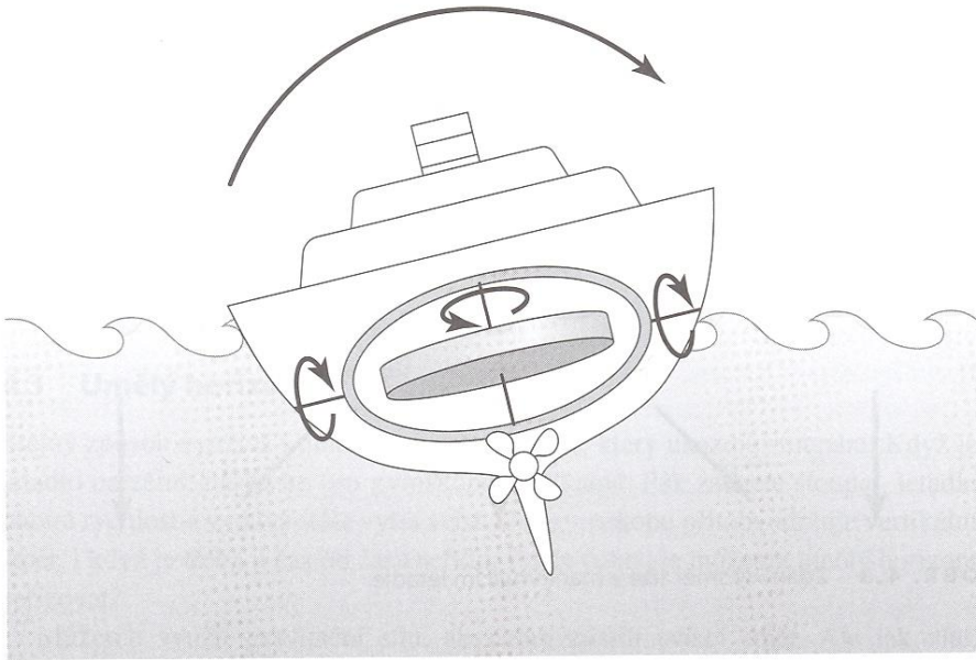
OBR. 4.4 Gyroskop ke stabilizaci lodi: zvedání gyroskopu dopředu vytváří silový moment, který nakloní loď do strany.
